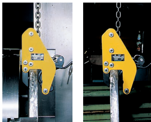
Pinza universale in esecuzione speciale con morsa piccola per l'utilizzo su macchine utensili.
