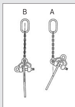
Sollevamento di grosse tubazioni in acciaio
